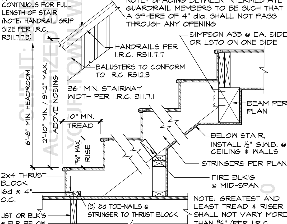
9 INTERIOR STAIR SCALE: 1" = 1'-0"
