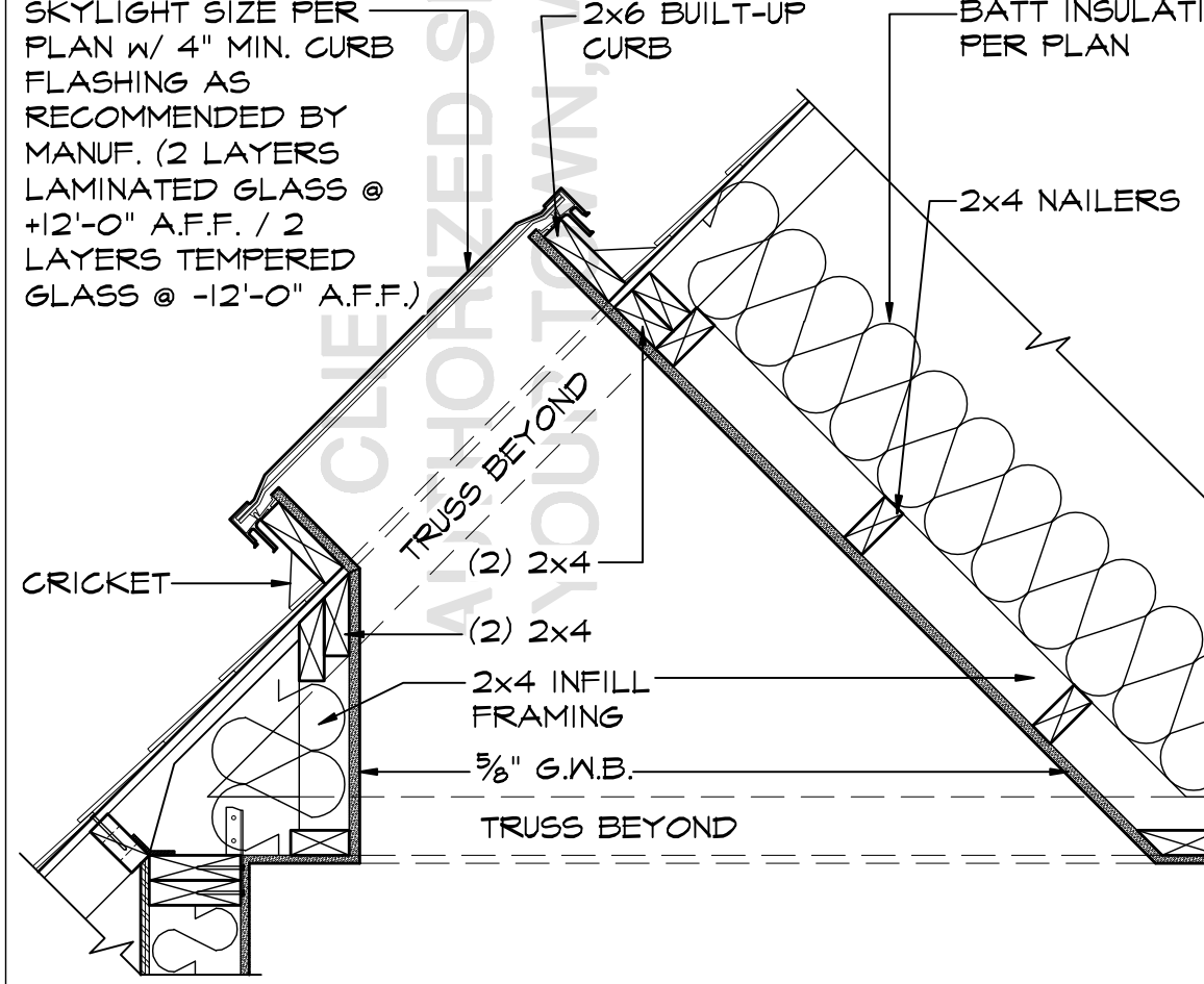
16 SKYLIGHT SCALE: 1" = 1'-0"
