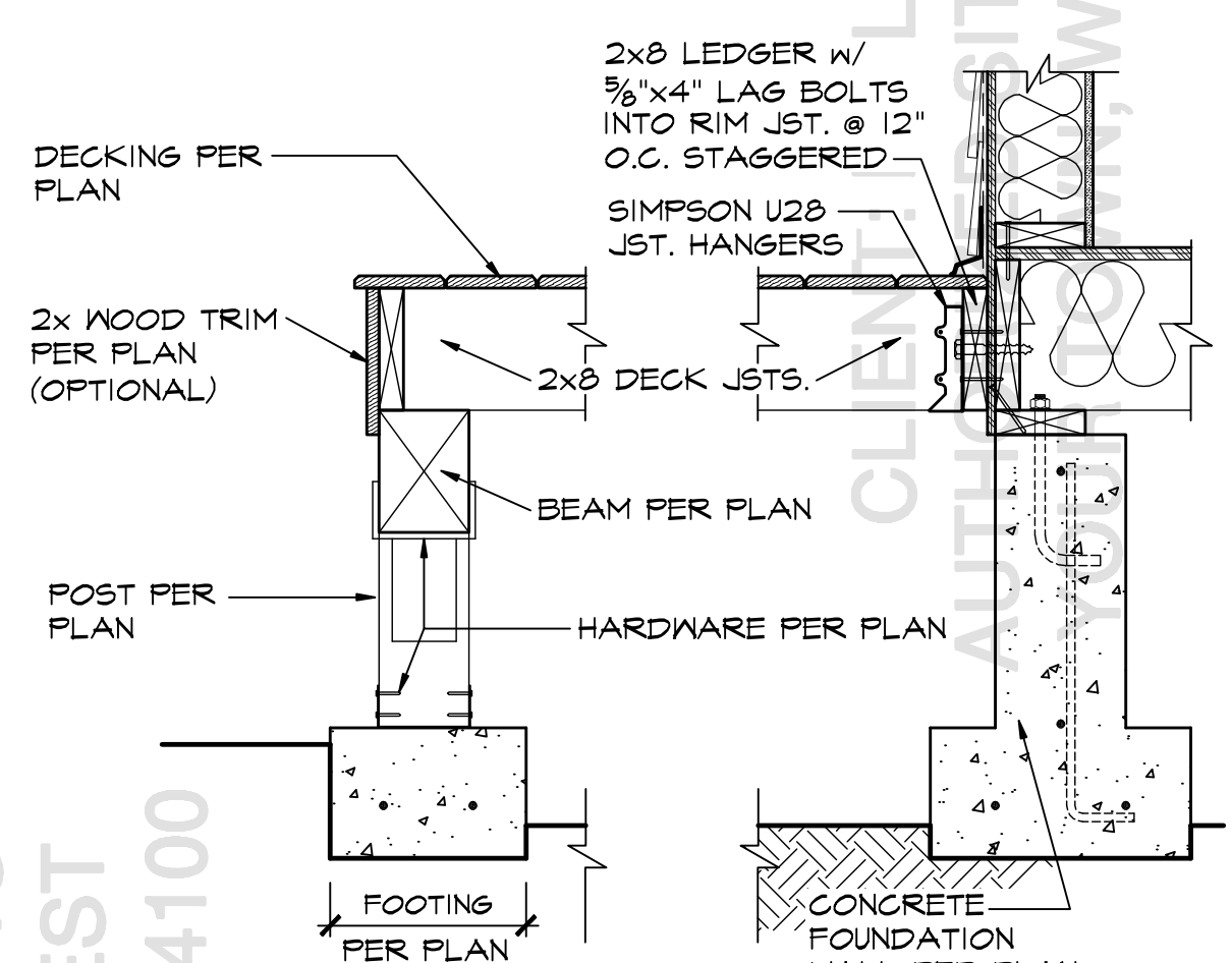
7 DECK SCALE: 1" = 1'-0"
