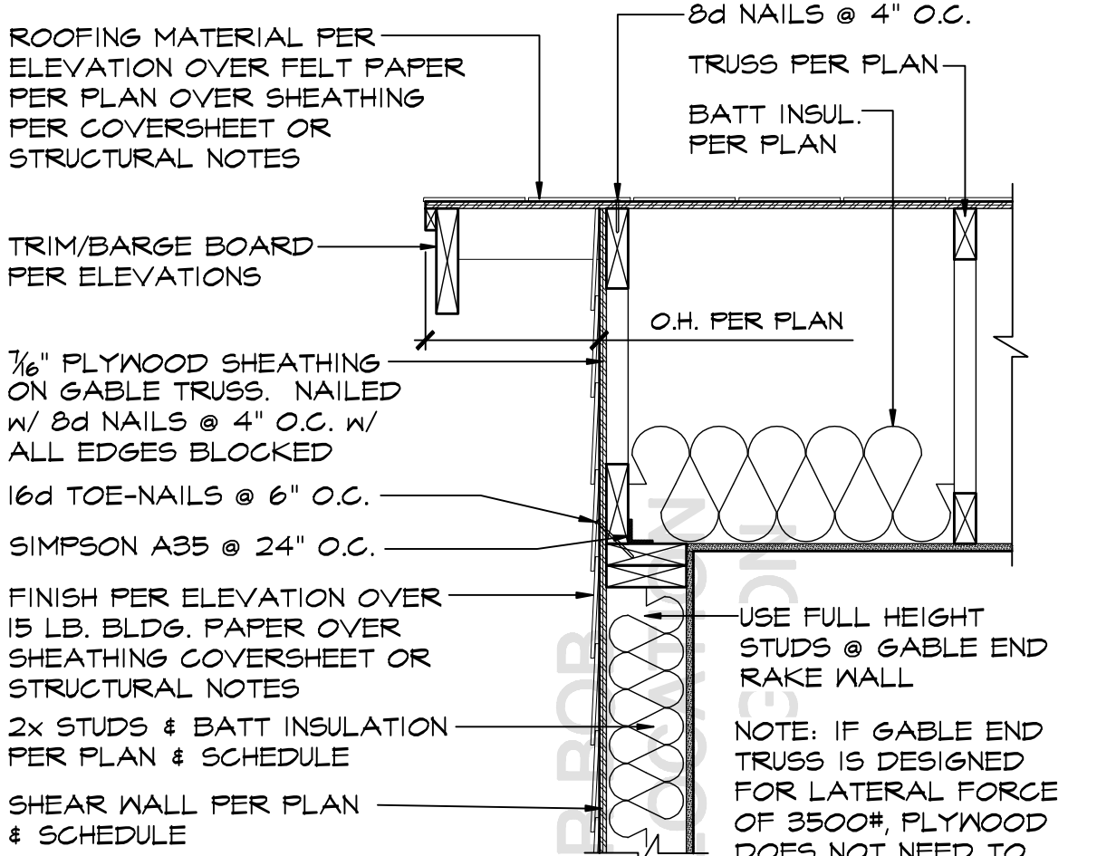
15 GABLE END DETAIL SCALE: 1" = 1'-0"
