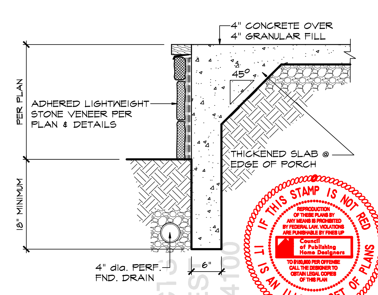
8 PORCH SCALE: 1" = 1'-0"
